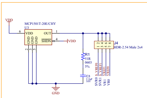
VREF Circuit
